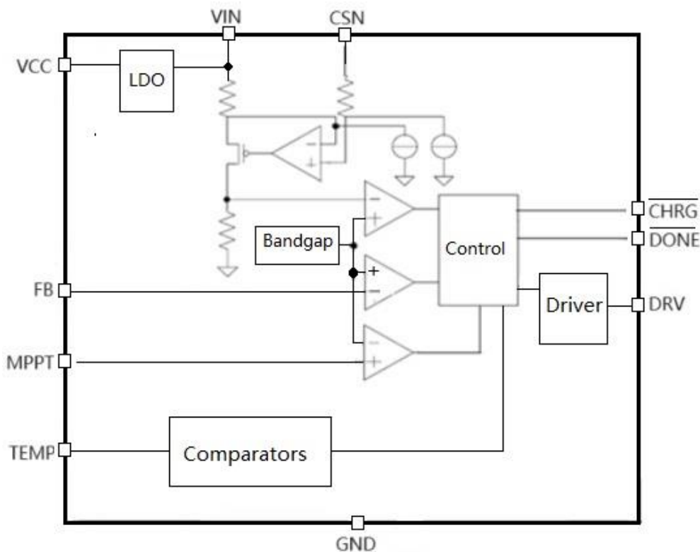
图 2 功能框图
